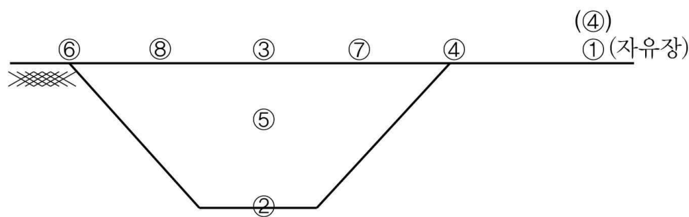
[별도 9] 일반적인 댐 및 저수지의 지진가속도감지기 설치 위치(제20조 관련)
